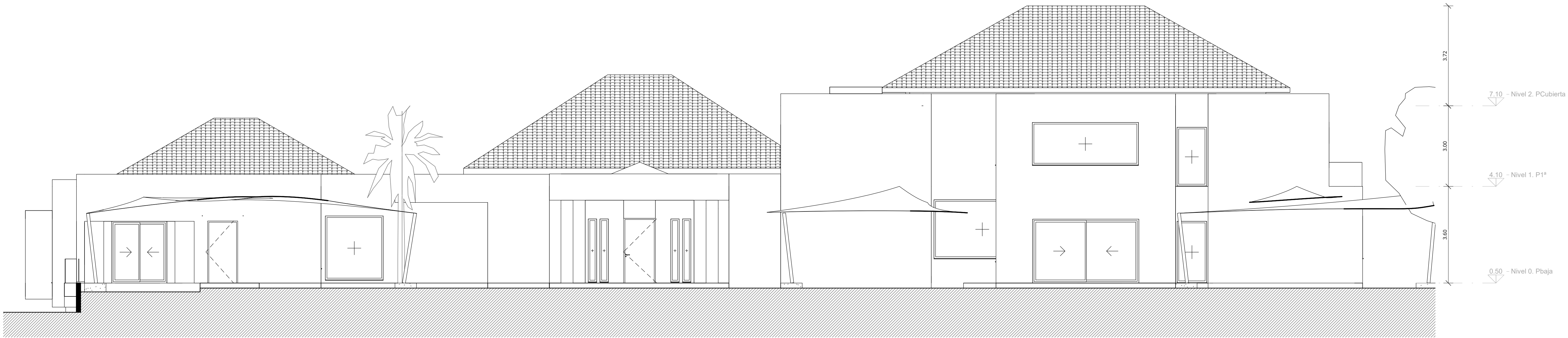
REFORMADO - Alzado Norte 1 : 75
